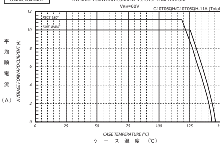
平均順電流 - ケース温度定格 AVERAGE FORWARD CURRENT - CASE TEMPERATURE
