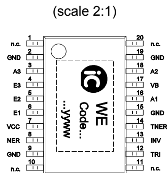
TSSOP20tp 4.4 mm
