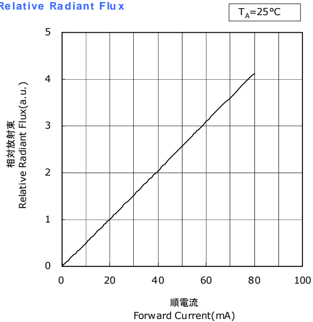
順電流-相対放射束特性
