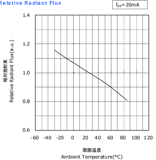
周囲温度-相対放射束特性
