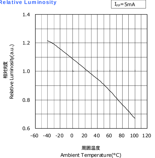
周囲温度-相対光度特性
