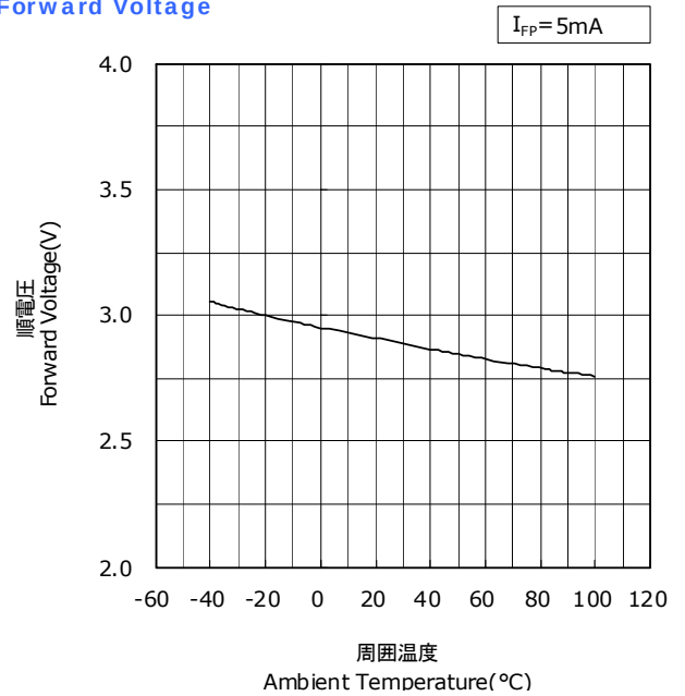
周囲温度-順電圧特性
