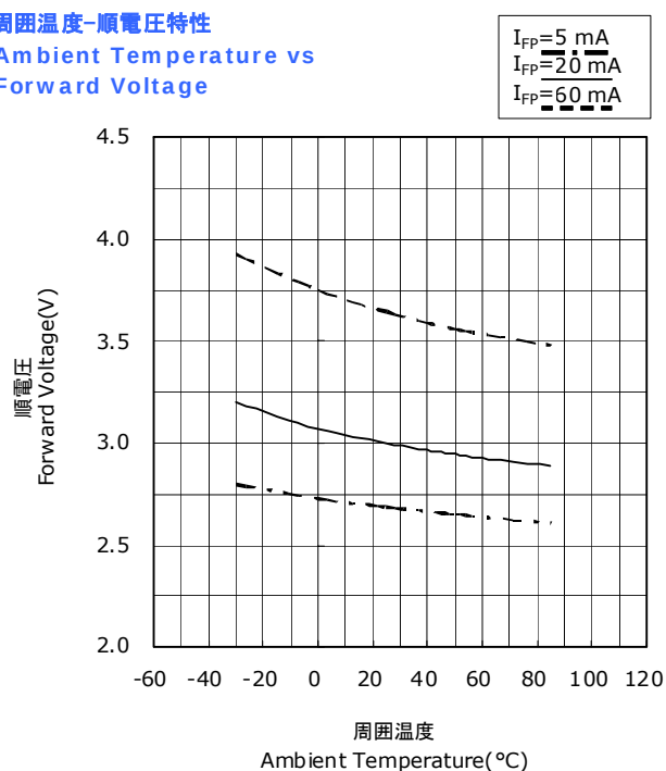
周囲温度-順電圧特性
