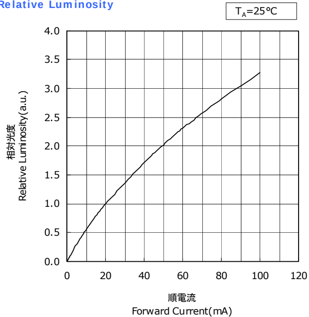
順電流-相対光度特性
