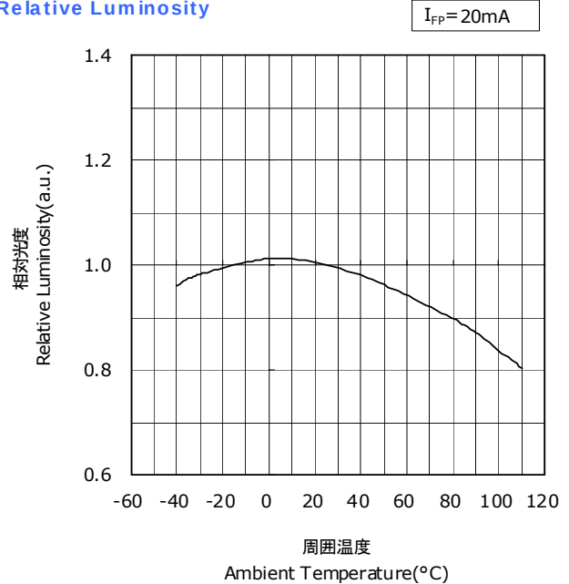
周囲温度-相対光度特性
