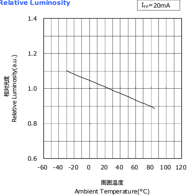
周囲温度-相対光度特性
