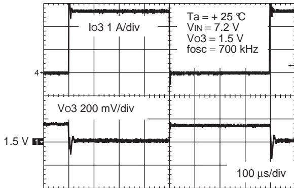
CH3 (Vo3 = 1.5 V) Io3 = 0 A ↔ 2.7 A, Io3 slew rate = 2.7 A/μs
