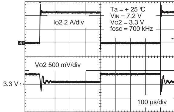
CH2 (Vo2 = 3.3 V) Io2 = 0 A ↔ 4.5 A, Io2 slew rate = 4.5 A/μs
