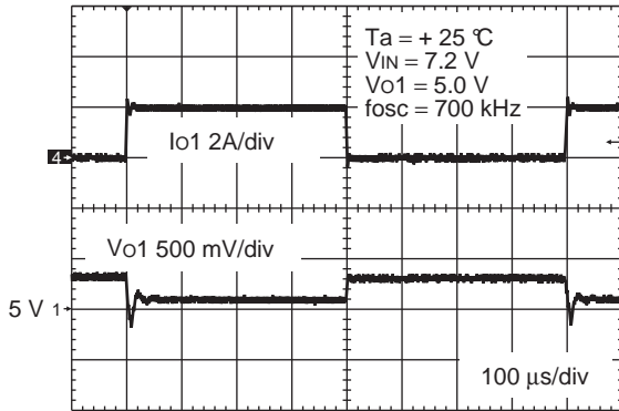
CH1 (Vo1 = 5.0 V) Io1 = 0 A ↔ 2 A, Io1 slew rate = 2 A/μs
