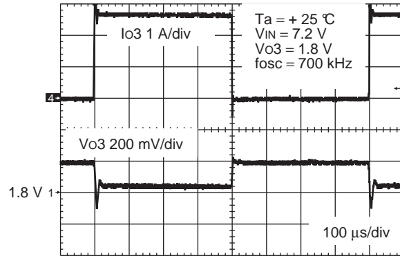
CH3 (Vo3 = 1.8 V) Io3 = 0 A ↔ 2.7 A, Io3 slew rate = 2.7 A/μs
