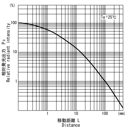
■相対発光出力／距離特性 P_0/L^{\times 1}
