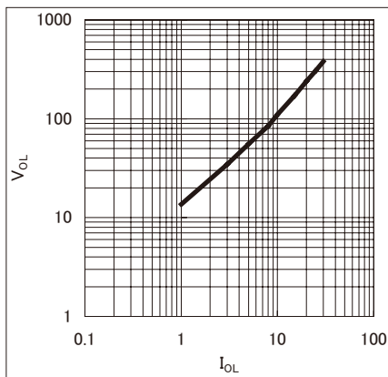
■ ローレベル出力電圧/ローレベル出力電流特性
