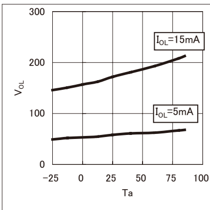
■ ローレベル出力電圧/周囲温度特性
