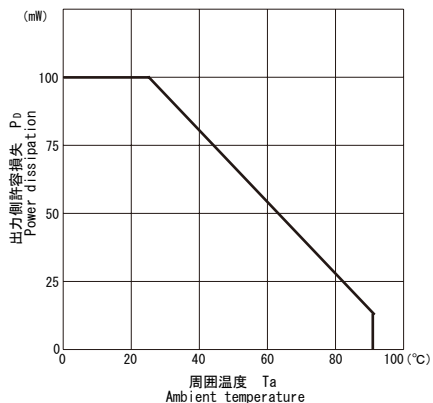
■出力側許容損失/周囲温度 P_b/T_a
