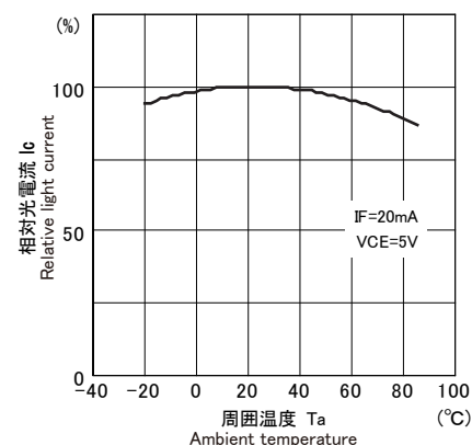
■相対光電流/周囲温度特性 I_c/T_a
