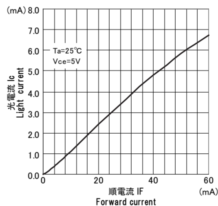
■順電流/光電流特性 I_c/I_f
