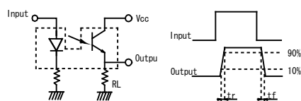
*1 応答時間測定回路
