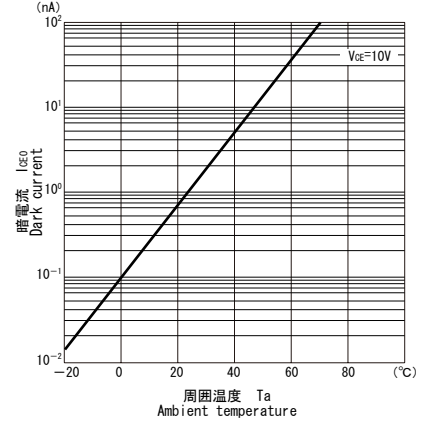
■暗電流/周囲温度特性 I_{CEO}/T_a
