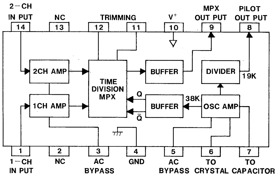
NJM2035D NJM2035M
