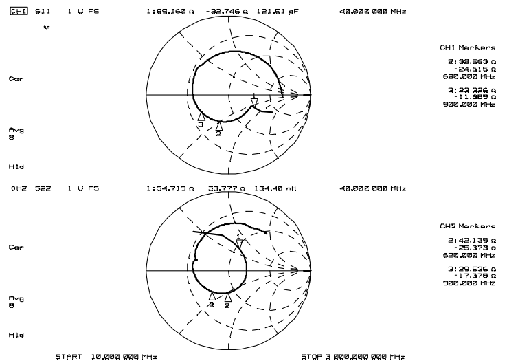
Zin, Zout (f=10MHz~3GHz)
