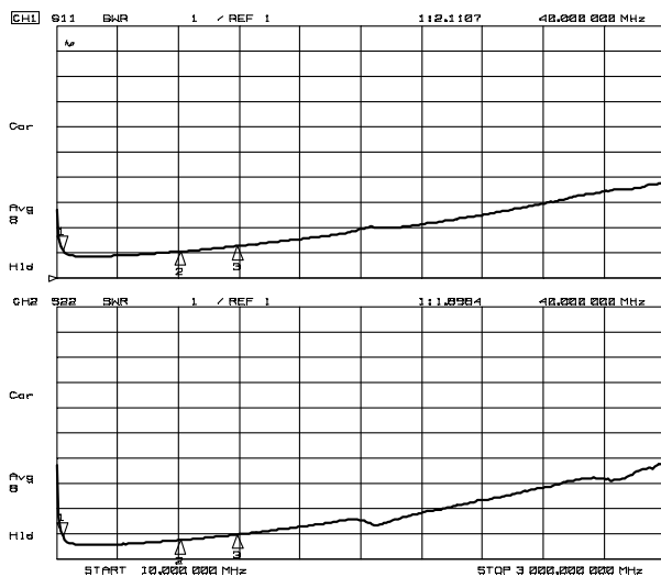
VSWR (f=10MHz~3GHz)
