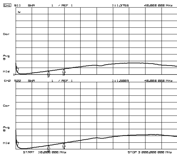
VSWR (f=10MHz~3GHz)
