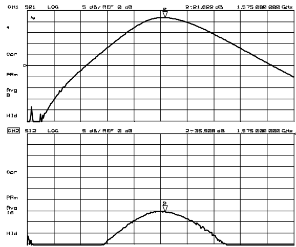
S21, S12
