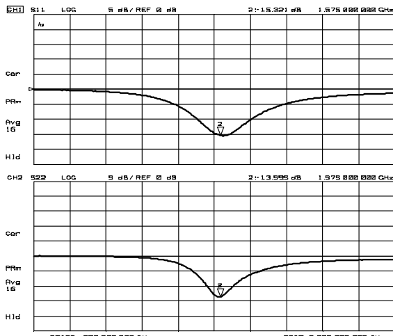
VSWR
