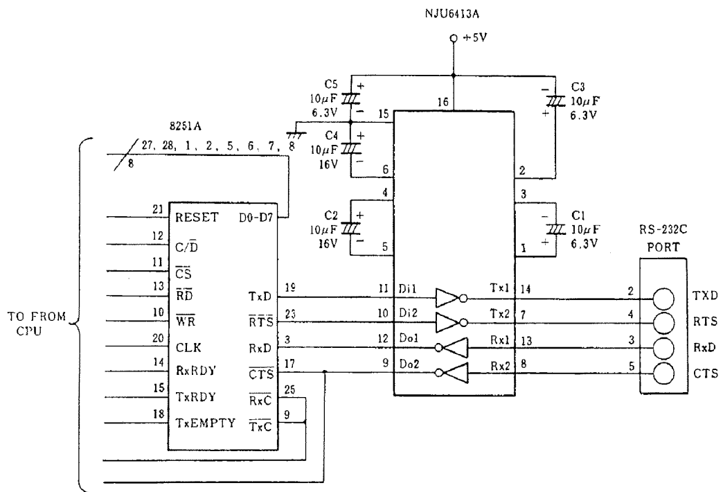
RS-232C port
