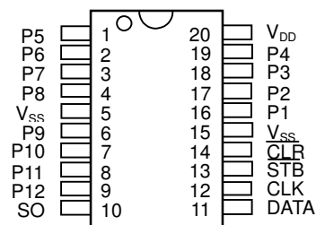
NJU3714AV
