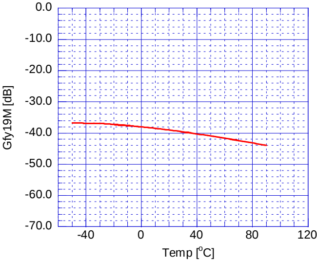
LPF19M vs Temp.
