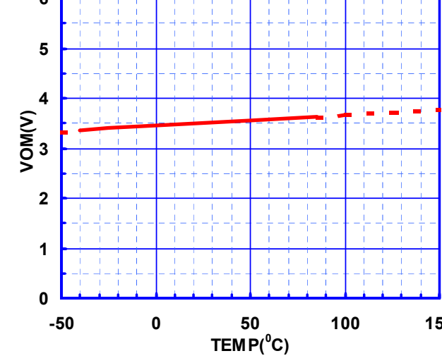
VOM vs Temperature (VINN)
