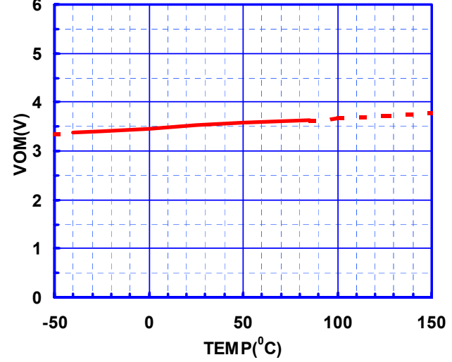
VOM vs Temperature (VINP)
