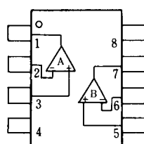
NJM2119D NJM2119M
