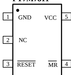
SOT23-5
