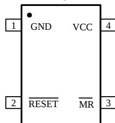
SOT143
