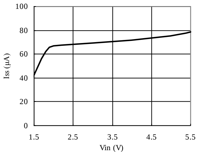
PT7M8220B (1.2V)
