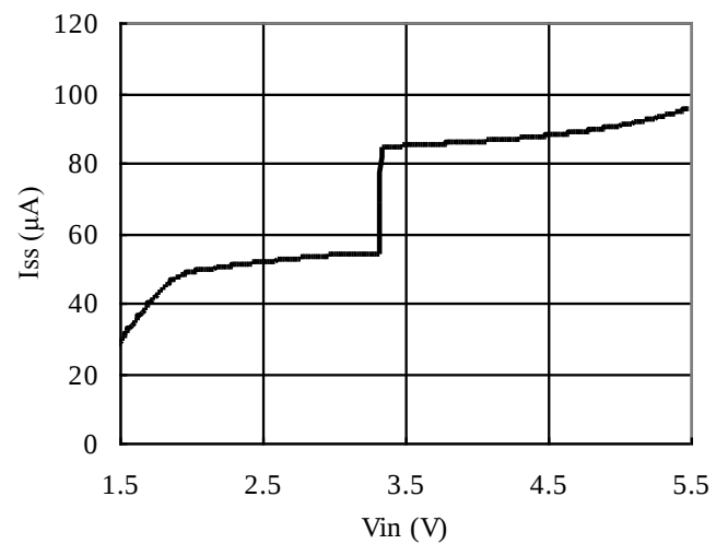
PT7M8220B (3.3V)
