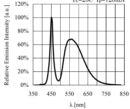
Spectrum T_c=25^\circ\text{C} I_F=720\text{mA}
