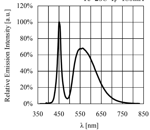
Spectrum T_c=25^\circ\text{C} I_F=180\text{mA}
