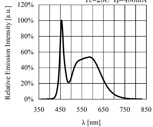
Spectrum T_c=25^\circ\text{C} I_F=480\text{mA}
