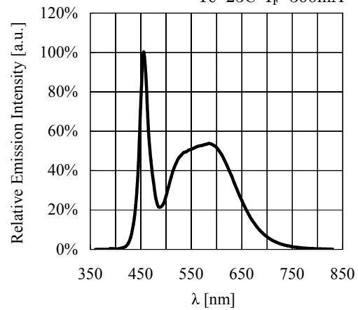
Spectrum T_c=25^\circ\text{C} I_F=300\text{mA}
