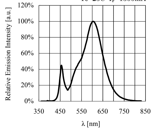
Spectrum T_c=25^\circ\text{C} I_F=1500\text{mA}
