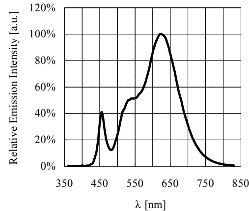
Spectrum T_c=25C , I_F=180\text{ mA}
