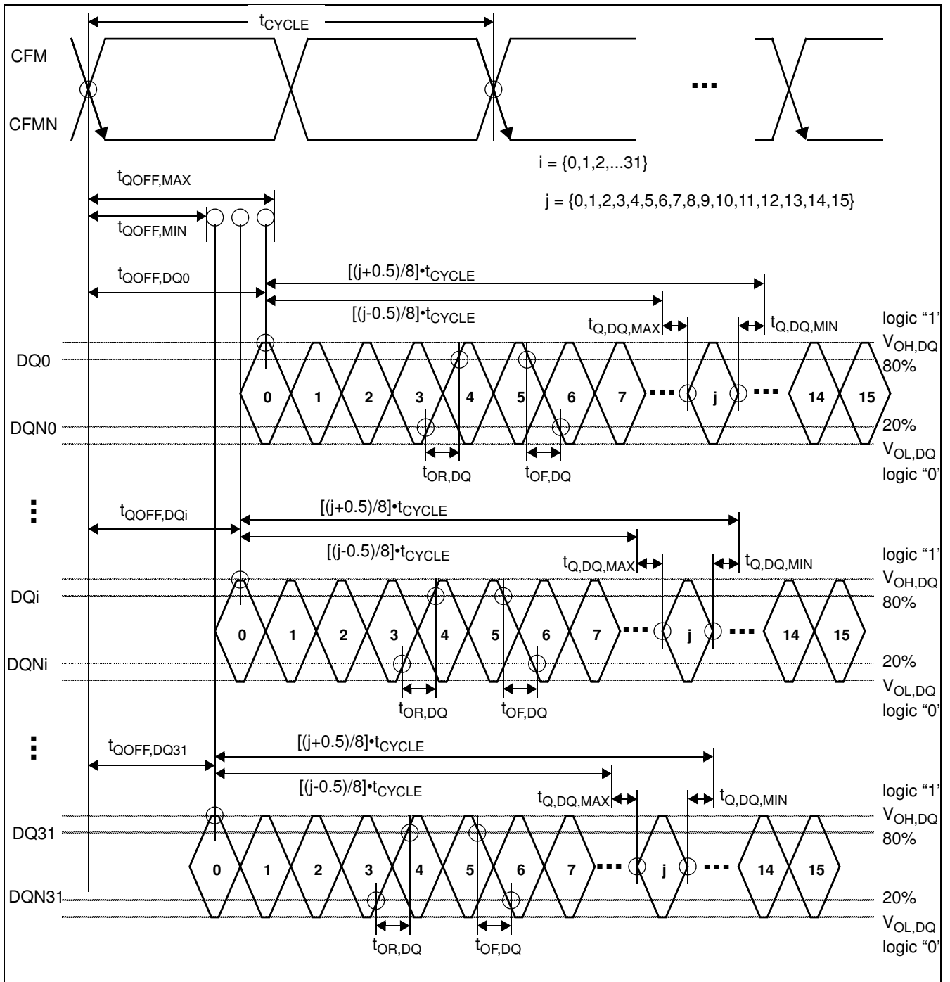
Figure 52 DRSL DQ Transmit Waveforms
