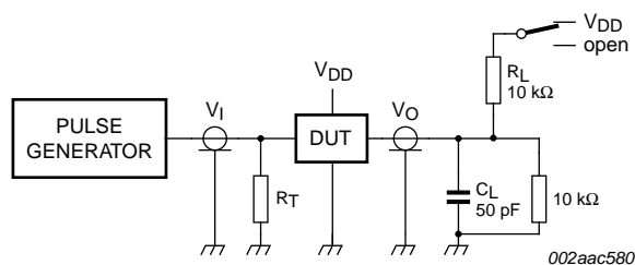
Fig 17. Test circuitry for enable/disable times, SDOUT ( t_{en}(SDOUT) and t_{dis}(SDOUT) )
