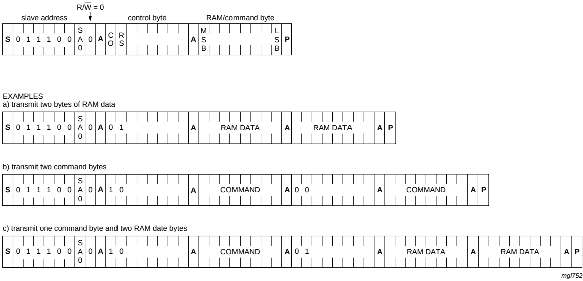
Fig 20. I 2 C-bus protocol
