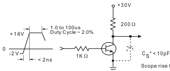
Fig. 1 Turn-On Time
