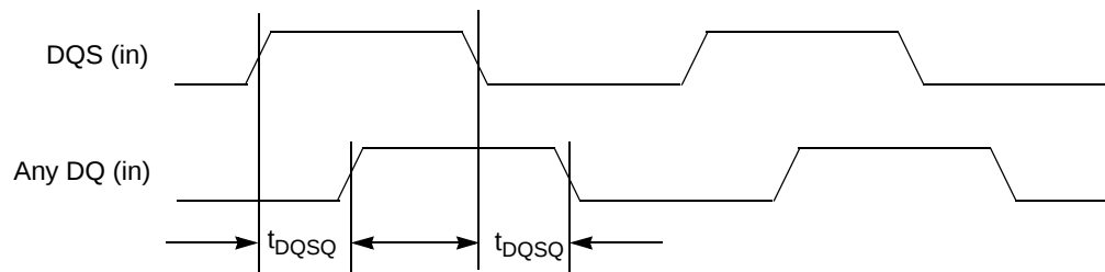
Figure 29. DDR read timing, DQ vs. DQS
