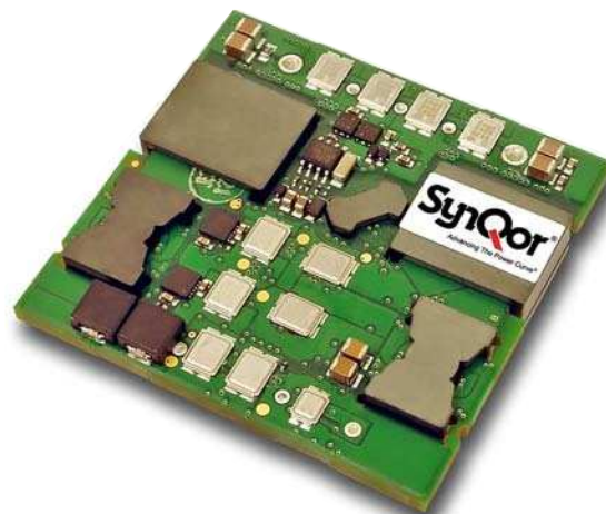
SQ60120HZA50 Module
