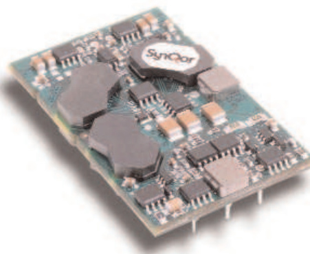
PQ60015QML15 Module
