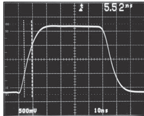
LT1187 • TPC23
