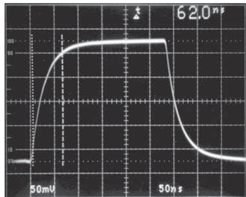
LT1187 • TPC25
