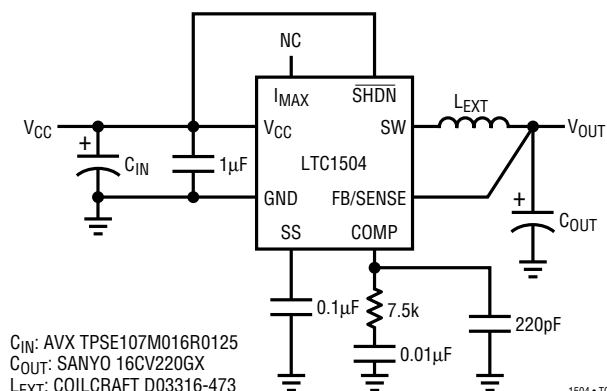
TEST CIRCUITS
