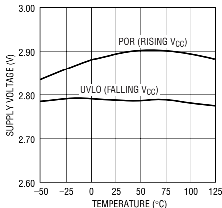
POR and UVLO vs Temperature
