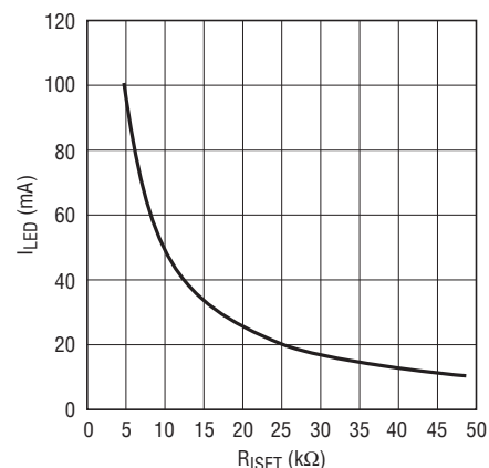
I_{\text{LED}} vs R_{\text{SET}}
