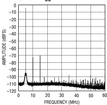
LTM9004-AD: 64k Point FFT
