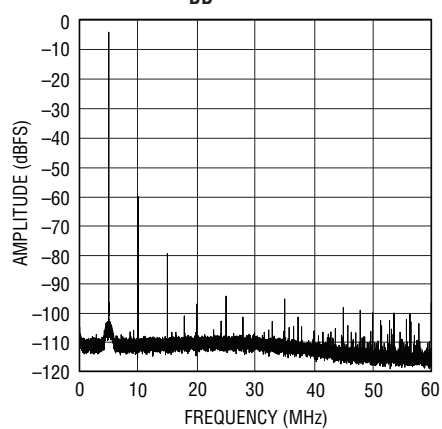
LTM9004-AD: 64k Point FFT
