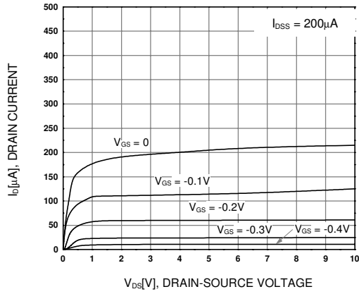
Figure 1. I_D - V_{DS}
