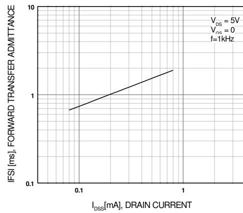
Figure 4. |y_{FS}| - I_{DSS}
