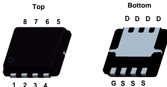
MLP 3.3x3.3
