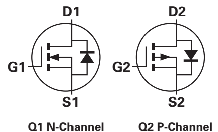
Q1 N-Channel
