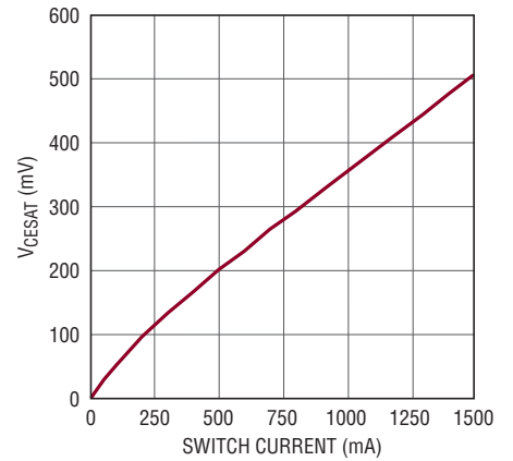
Switch V_{CESAT}
