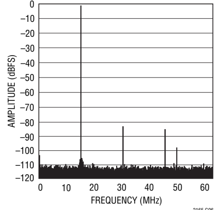
LTC2165 64k Point FFT, f_{IN} = 140\text{MHz} , -1\text{dBFS} , 125\text{Mps}
