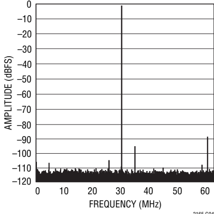
LTC2165 64k Point FFT, f_{IN} = 30\text{MHz} , -1\text{dBFS} , 125\text{Mps}
