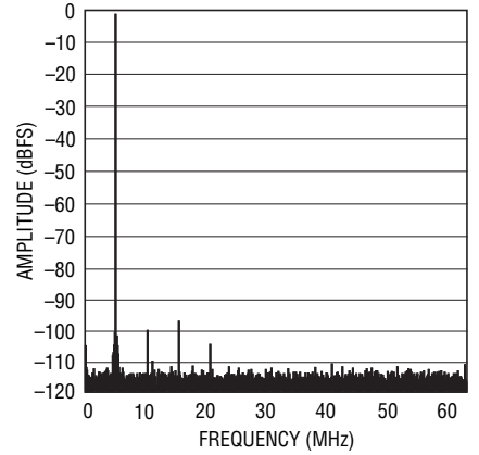
LTC2165 64k Point FFT, f_{IN} = 5\text{MHz} , -1\text{dBFS} , 125\text{Mps}
