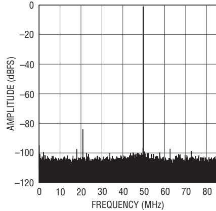
LTC2150-12: 32K Point FFT, f_{IN} = 121\text{MHz} , -1\text{dBFS} , 170\text{Mps}
