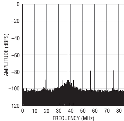
LTC2150-12: 32K Point FFT, f_{IN} = 380\text{MHz} , -1\text{dBFS} , 170\text{Mps}
