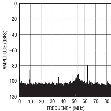
LTC2150-12: 32K Point FFT, f_{IN} = 225\text{MHz} , -1\text{dBFS} , 170\text{Mps}
