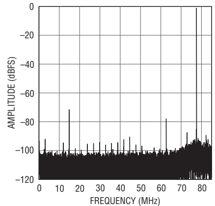
LTC2150-12: 32K Point FFT, f_{IN} = 420\text{MHz} , -1\text{dBFS} , 170\text{Mps}
