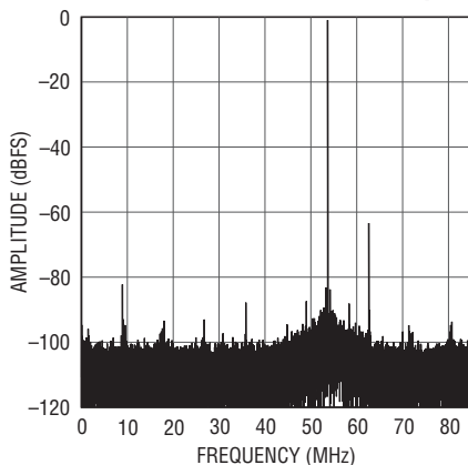
LTC2150-12: 32K Point FFT, f_{IN} = 567\text{MHz} , -1\text{dBFS} , 170\text{Mps}
