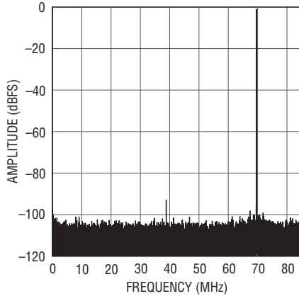
LTC2150-12: 32K Point FFT, f_{IN} = 70\text{MHz} , -1\text{dBFS} , 170\text{Mps}
