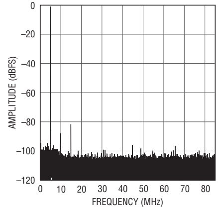
LTC2150-12: 32K Point FFT, f_{IN} = 176\text{MHz} , -1\text{dBFS} , 170\text{Mps}
