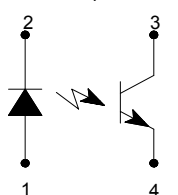
OPI7320, OPI7340
