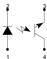
OPI7320RCE, OPI7340RCE
