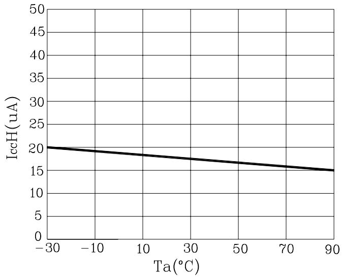
Fig. 3 I_{CCH} - T_a
