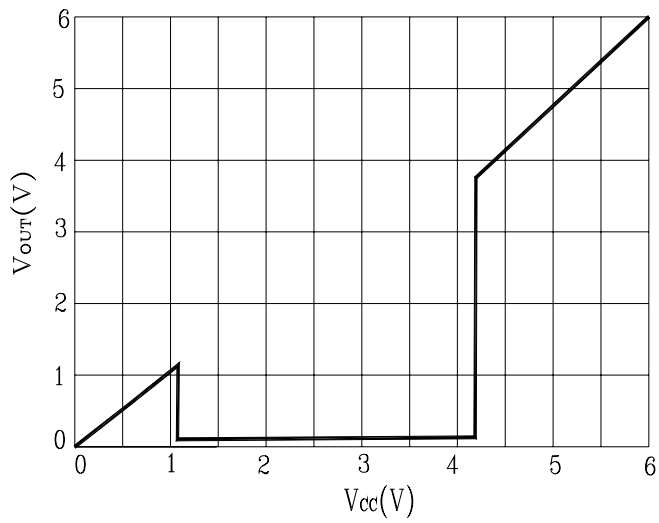
Fig. 1 V_{OUT} - V_{CC}
